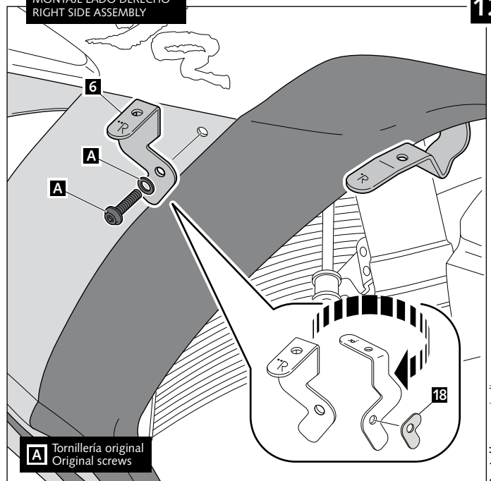
MONTAJE LADO DERECHO RIGHT SIDE ASSEMBLY
